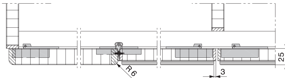
Türen vorliegend
