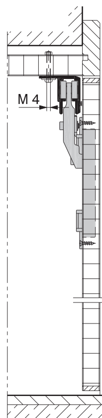
Puertas enrasadas
