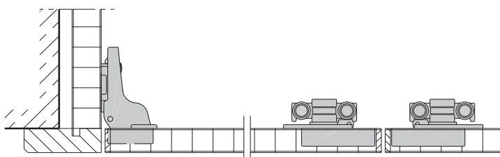
Puertas superpuestas
