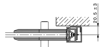
Montage devant le mur
