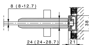
Montage mural
