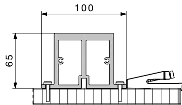
Profil vormontiert
