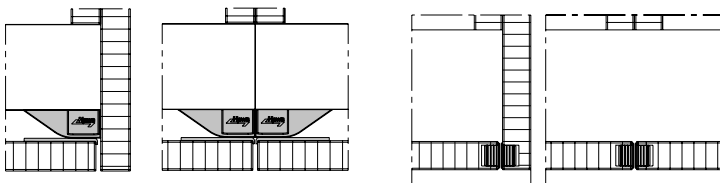
Flächenbündige Türpositionierung mit Bodenprofil und Auflauframpe
